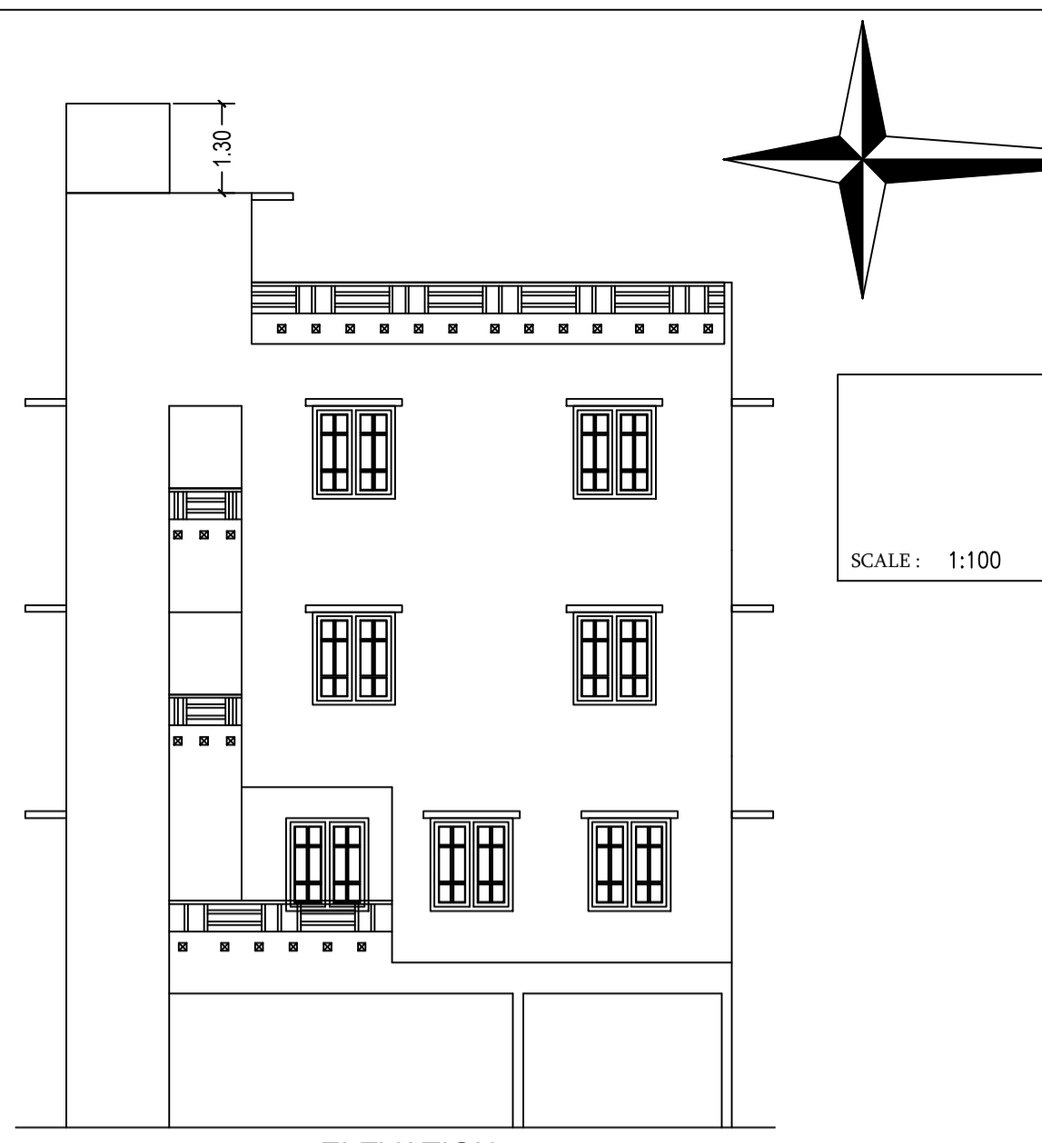
ELEVATION
